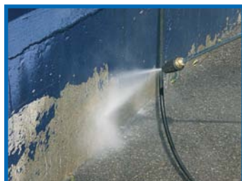
Festékel távolítás turbófúvókával
